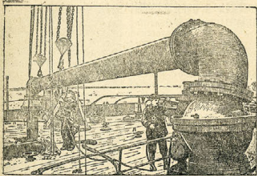
На снимке: Перекачка топкого мазута из баржи. Рис. с фото Н. Борисова („Прессклише“).
