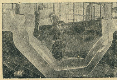
Из снимков: Одна из частей изложницы весом 82 тонны обрабатываемая в механическом цехе. Фото И. Водянова.
