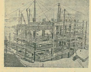
Первые стальные конструкции металлического каркаса нижней части здания Дворца Советов. Фото Г. Широкова. Фото-книжка ТАСС.
